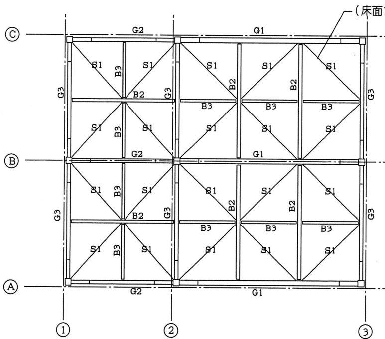
R階伏図 1:100
