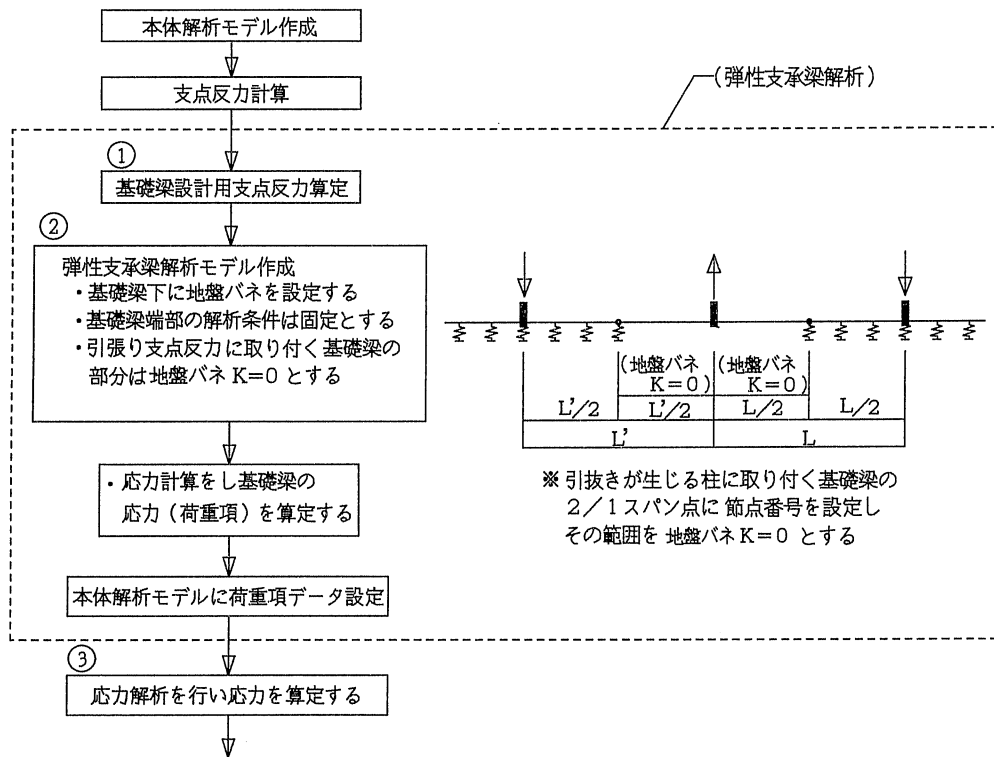
[弾性支承梁解析 フロー図]
