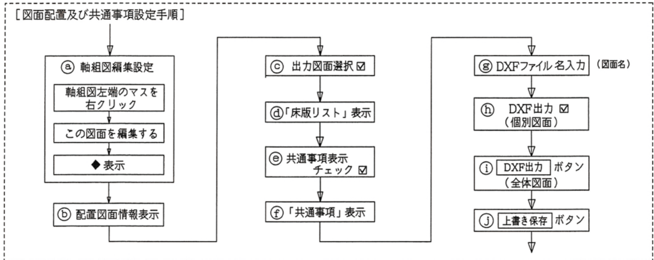
[ 図面配置 ] ダイアログ
